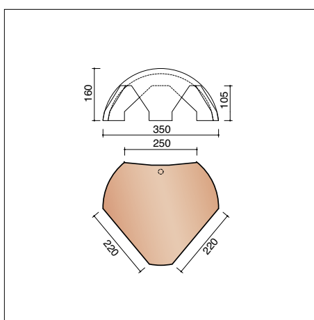
M0005870 Jonction en combinaison avec faîtières angulaires 1900/2800 (3 directions)
