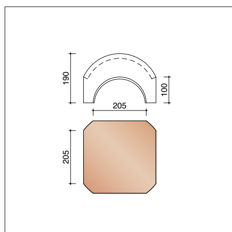
M0005610 Jonction en combinaison avec faîtières angulaires 1900/2800 (4 directions)
