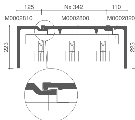
PLAN DE POSE TRANSVERSALE DE LA TOITURE AU NIVEAU DE LA FAÎTIÈRE ANGULAIRE ACTUA
