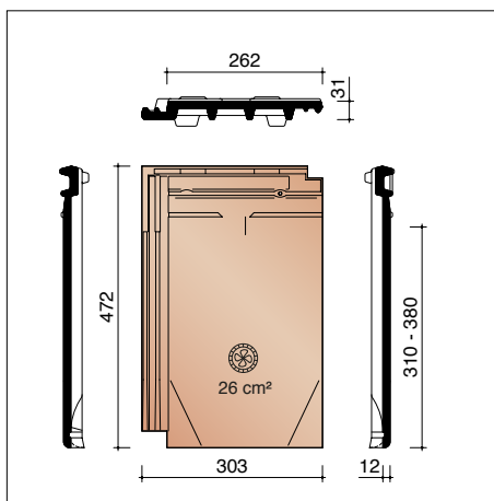
MACT8640 Tuile châtière avec grille synthétique - 26 cm²
