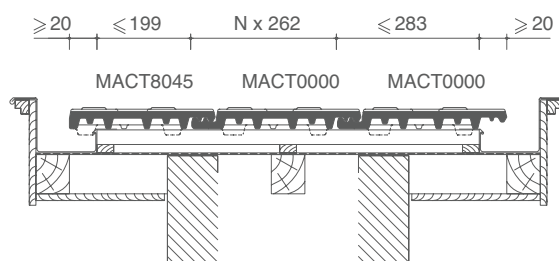
PLAN DE POSE TRANSVERSALE DE LA TOITURE AU NIVEAU DE LA TUILE SANS EMBOÎTEMENT
