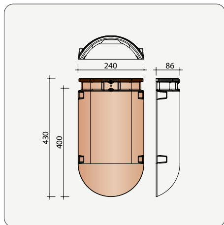
B0001260 About d'arêtier demi-rond Pour la couleur Rouge naturel
