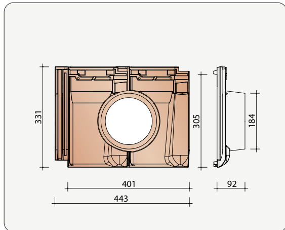
BCFL8749 Tuile à douille Ø 150 mm
