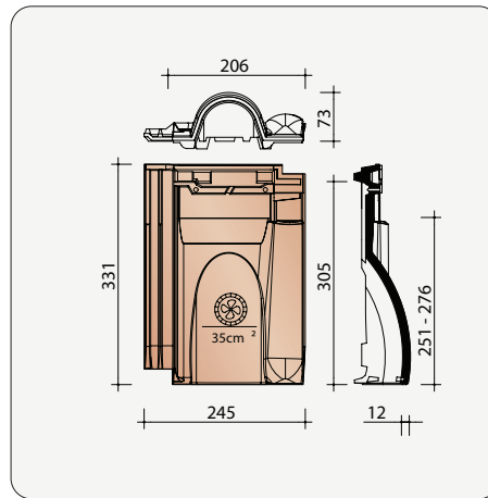
BCFL8640 Tuile châtière avec grille - 35 cm 2
