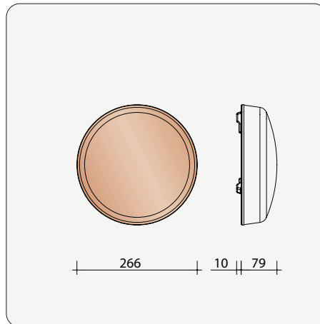
BCFL8721 Mitron d'aérage pour tuile à douille Ø 100/150 mm
