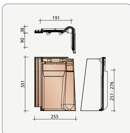
BCFL7090 3,6 pièces/m crt Tuile de rive droite
