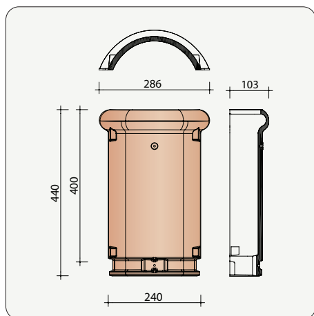
B0001200 2,5 pièces/m crt Faîtière demi-ronde - arêtier Pour la couleur Rouge naturel
