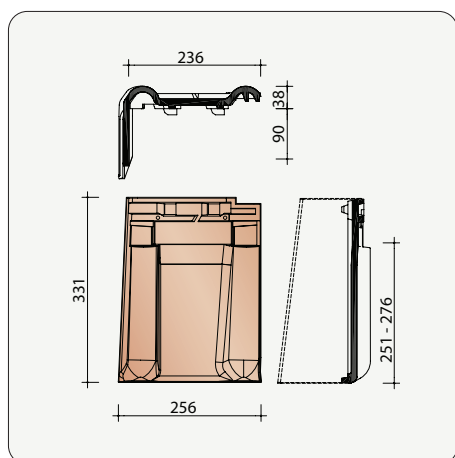
BCFL7080 3,6 pièces/m crt Tuile de rive gauche
