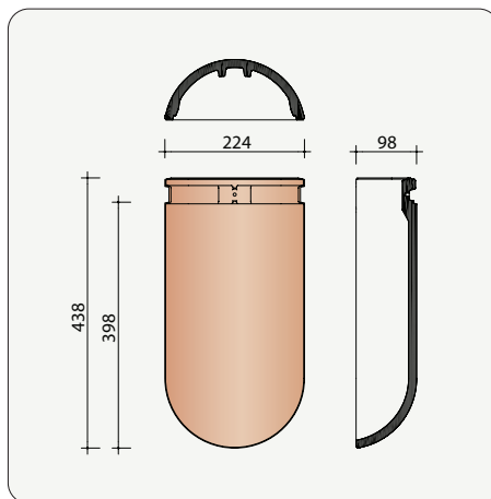
B0001260 About d'arêtier demi-rond Pour les couleurs Rouge flammé et Ardoisé
