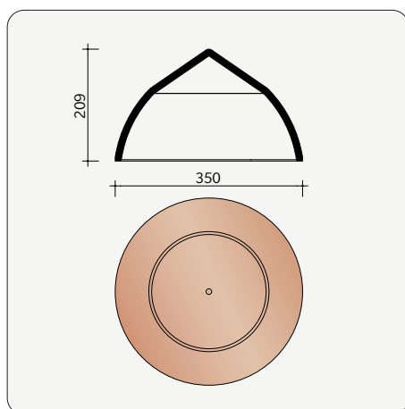
B0005324 Jonction sans découpes
