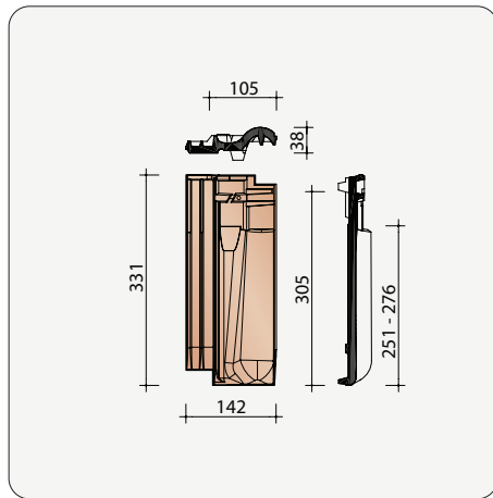
BCFL8010 3,6 stuks/lm Halve pan
