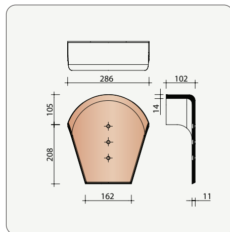
B0001240 Kopplaat voor halfronde vorst
