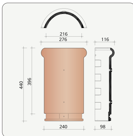
B0001200 2,5 stuks/lm Halfronde vorst - noordboom Voor de kleuren Rood gevamd en Antraciet mat
