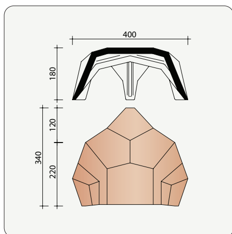
G0005870 Jonction PD pour 1 faîtière et 2 arêtiers
