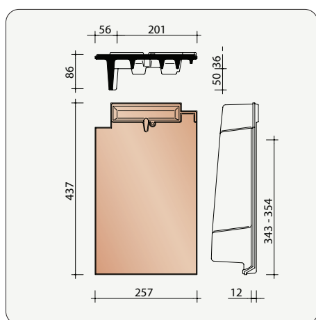
GDOM7081 2,9 pièces/m crt Tuile de rive gauche modèle allemand
