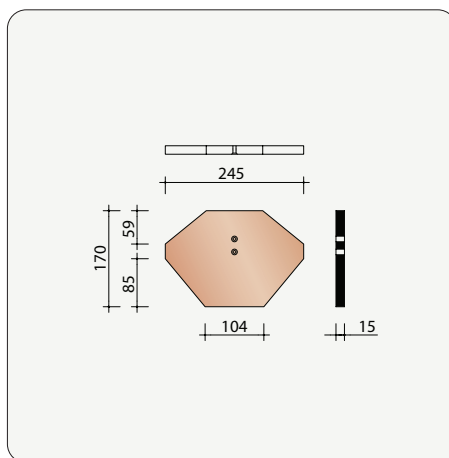
G0002840 Fronton pour faîtière angulaire PD
