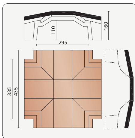
G0005871 Jonction PD pour 4 arêtiers
