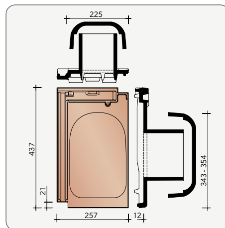
GDOM8728 Kit tuile à douille Ø 125 mm + mitron + adaptateur sous-toiture
