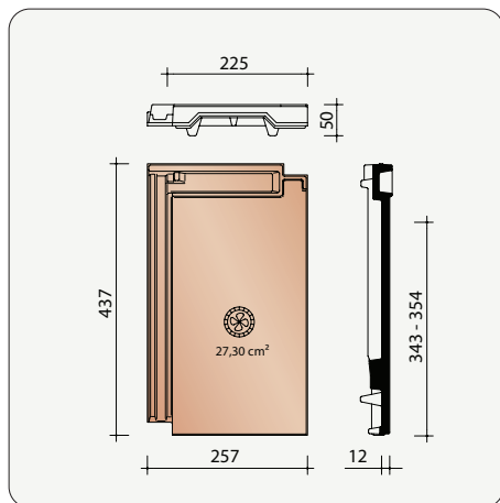
GDOM8610 Tuile châtère - 27,3 cm²
