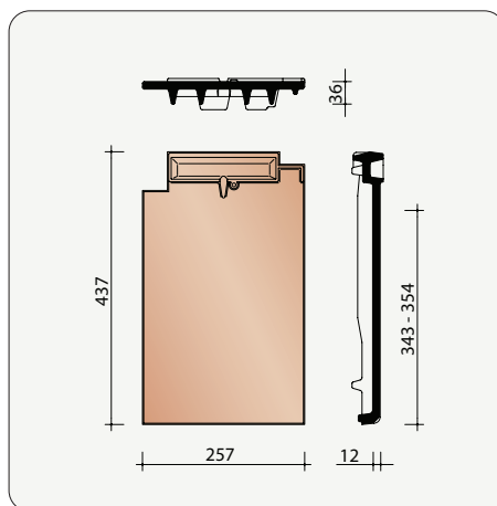
GDOM8045 2,9 pièces/m crt Tuile sans emboîtement
