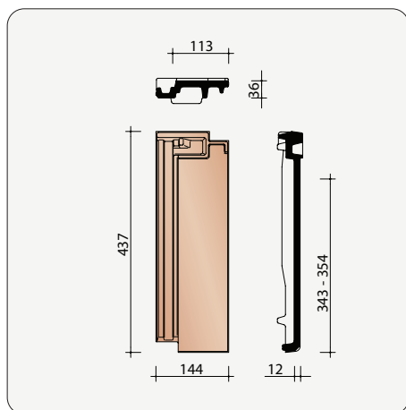
GDOM8010 1,45 pièces/m crt joints croisés Demi-tuile 2,9 pièces/m crt joints droits
