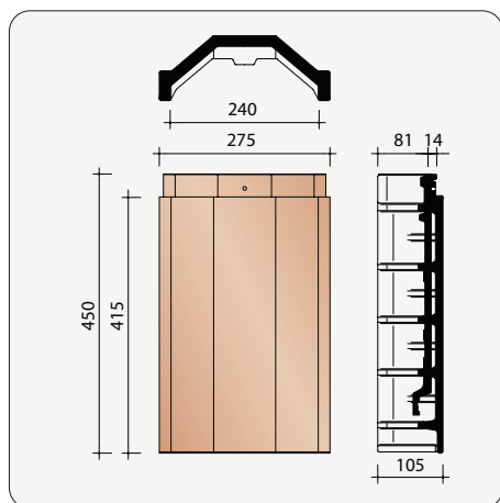
G0002800 2,5 pièces/m crt Faîtière angulaire - Arêtier PD
