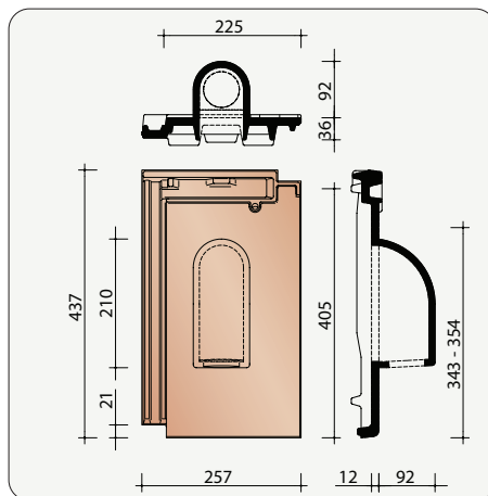
GDOM8958 Tuile de passage pour tuyau (Solar) + adaptateur sous-toiture
