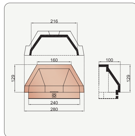
G0002860 About d'arêtier angulaire PD
