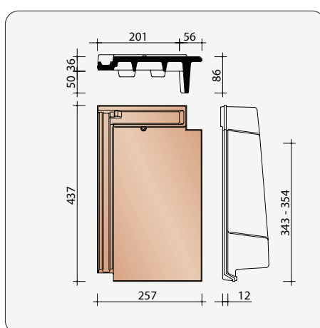
GDOM7091 2,9 pièces/m crt Tuile de rive droite modèle allemand
