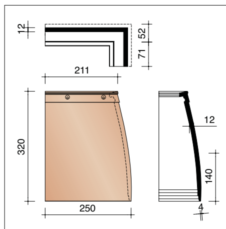
PELF8810 3,6 stuks/lm Rechter hoekstuk (gevelbekleding)
