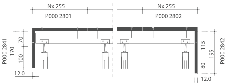
DWARSDOORSNEDE DAK TER HOOGTE VAN DE VORST 30° EN VAN DE VORST 45°
