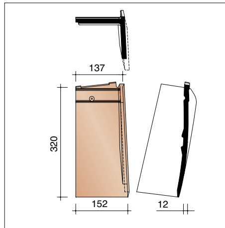
PELF7130 3,6 stuks/lm Speciale rechter halve gevelpan
