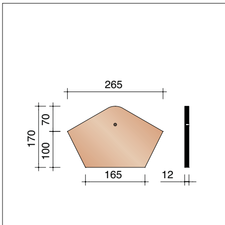
P0002841 Kopplaat voor hoekige vorst zonder sluiting 30°
