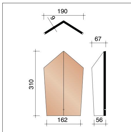
P0003711 Kleine hoekige beginnoordboom
