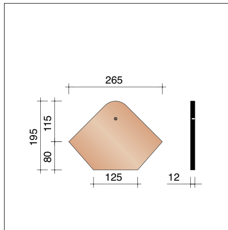
P0002842 Kopplaat voor hoekige vorst zonder sluiting 45°
