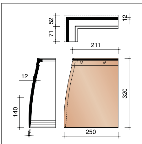
PELF8800 3,6 stuks/lm Linker hoekstuk (gevelbekleding)
