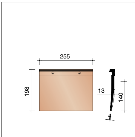
PELF8110 4 stuks/lm Korte pan
