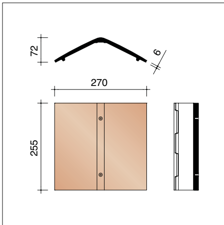
P0002801 4 stuks/lm Hoekige vorst zonder sluiting 30°
