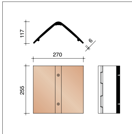
P0002802 4 stuks/lm Hoekige vorst zonder sluiting 45°
