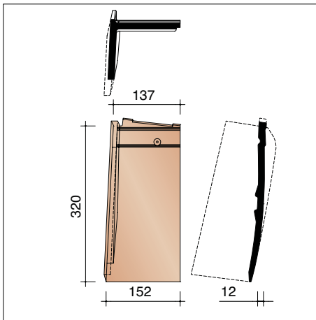
PELF7120 3,6 stuks/lm Speciale linker halve gevelpan
