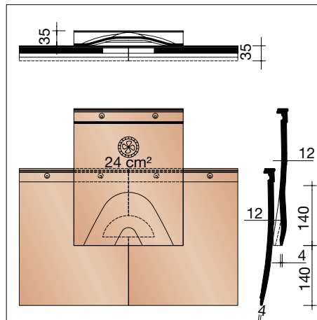
PELF8611 Kit ventilatiepan met rooster - 24 cm 2
