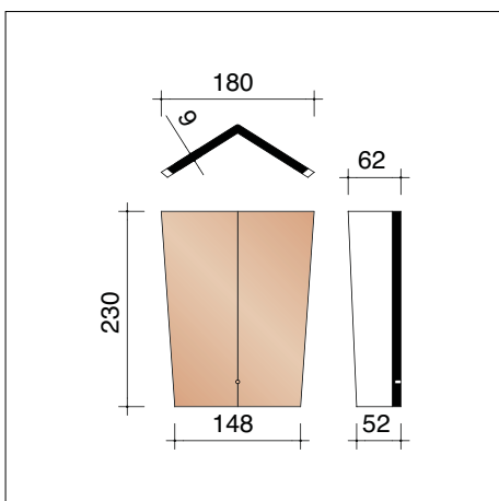
P0003701 6 stuks/lm Kleine hoekige noordboom
