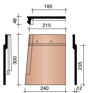
P0007070 RIVE INDIVIDUELLE DROITE POUR SARKING
