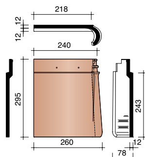
P0007060 RIVE INDIVIDUELLE GAUCHE POUR SARKING
