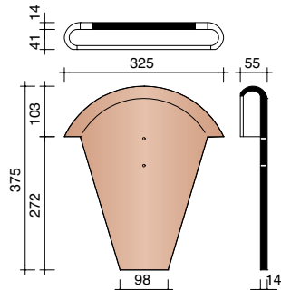
P0001241 FRONTON POUR SARKING
