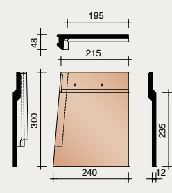
P0007071 RECHTER GEVELPLAAT SARKING VOOR STORMPAN 44 & 993
