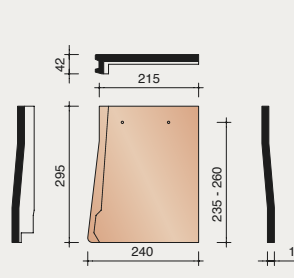
PVAR7071 RECHTER GEVELPLAAT SARKING VOOR STORMPAN VARIO 18
