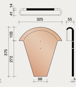
P0001241 KOPPLAAT SARKING VOOR ALLE STORMPANNEN
