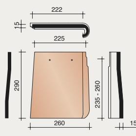
PVAR7061 LINKER GEVELPLAAT SARKING VOOR STORMPAN VARIO 18
