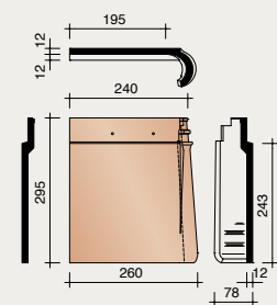
P0007061 LINKER GEVELPLAAT SARKING VOOR STORMPAN 44 & 993
