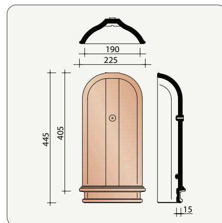
H0001360 About d'arêtier pour faîtière plate PH
