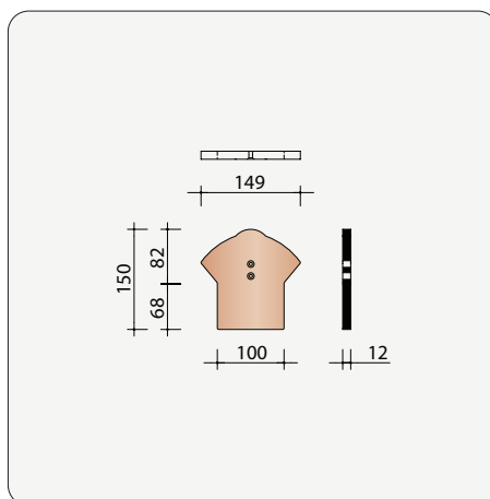
H0001340 Fronton pour faîtière plate PH
