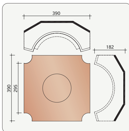
H0005240 Jonction W2 PV/PH/PI pour 4 arêtières
