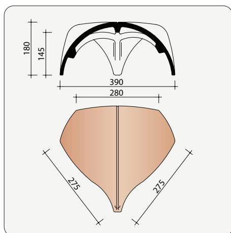
H0005230 Jonction W2 PV/PH/PI pour 1 faitière et 2 arêtières
