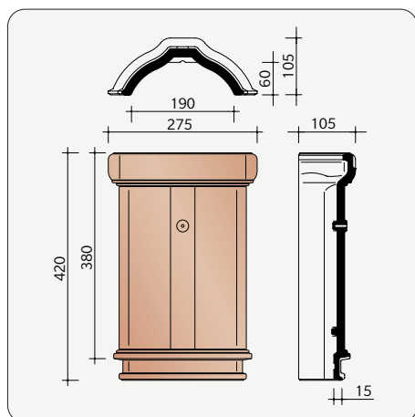
H0001300 2,6 pièces/m crt Faîtière plate - Arêtier PH
