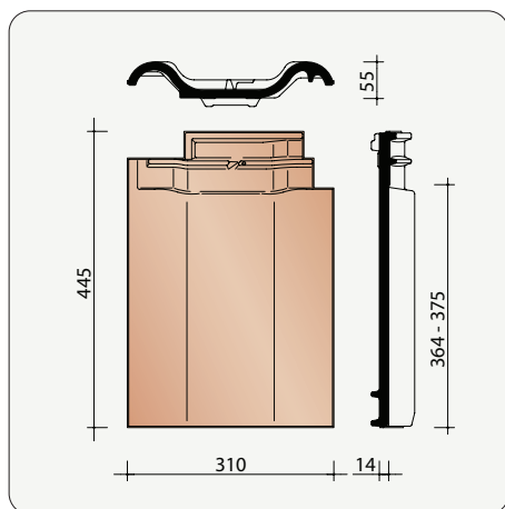
HHAR8050 2,7 pièces/m crt Tuile à double bourrelet
