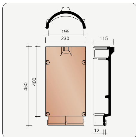
H0001001 2,5 pièces/m crt Faîtière demi-rond - Arêtier PV
