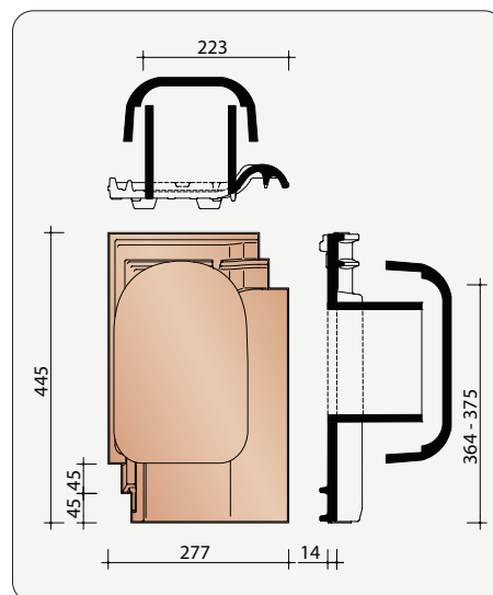
HHAR8728 Kit tuile à douille Ø 125 mm + mitron + adaptateur sous-toiture
