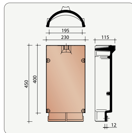
H0001071 About d'arêtier demi-rond PV
