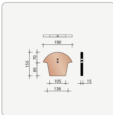
H0001041 Fronton pour faîtière demi-ronde PV
