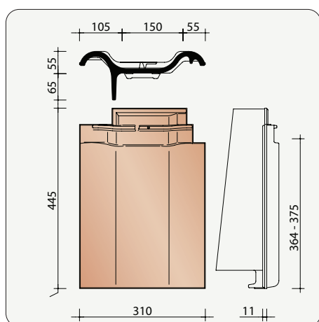
HHAR7081 2,7 pièces/m crt Tuile de rive gauche modèle allemand
