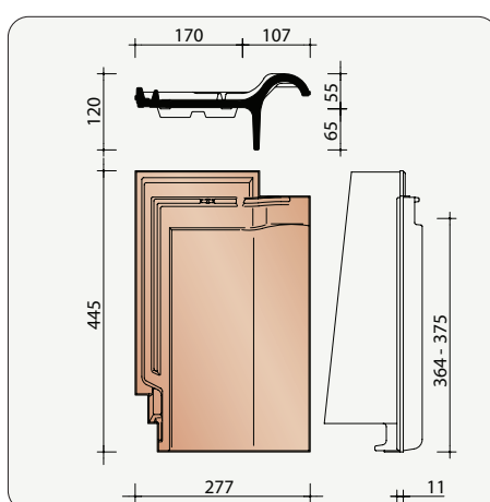
HHAR7091 2,7 pièces/m crt Tuile de rive droite modèle allemand
