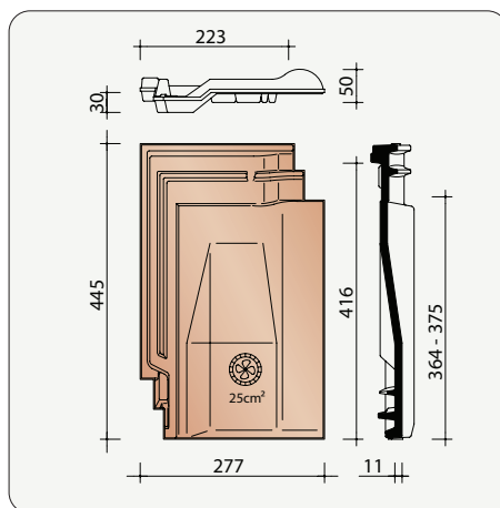
HHAR8610 Ventilatiepan - 25 cm 2
