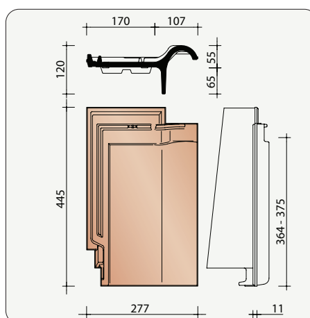
HHAR7091 2,7 stuks/lm Rechter gevelpan Duits model
