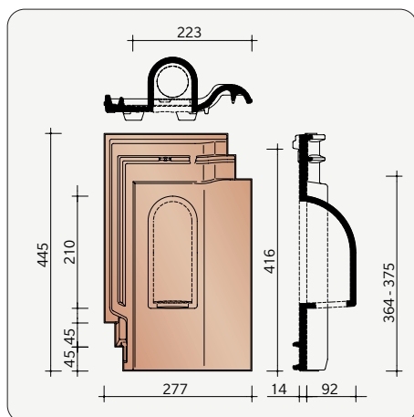
HHAR8958 Kabeldoorvoerpan (Solar) + onderdakadapter
