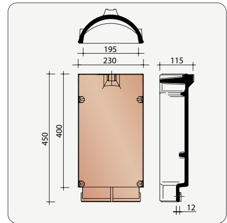
H0001071 Halfronde beginnoordboom PV
