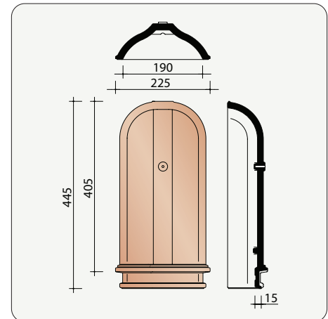
H0001360 Beginnoordboom voor platte vorst PH
