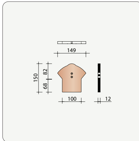
H0001340 Kopplaat voor platte vorst PH
