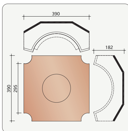
H0005240 Vorstenhoed W2 PV/PH/PI voor 4 noordbomen
