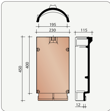
H0001001 2,5 stuks/lm Halfronde vorst - Noordboom PV
