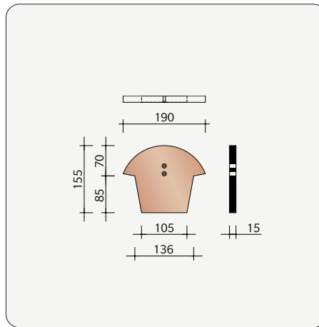
H0001041 Kopplaat voor halfronde vorst PV
