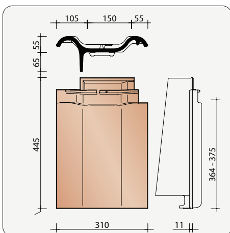
HHAR7081 2,7 stuks/lm Linker gevelpan Duits model
