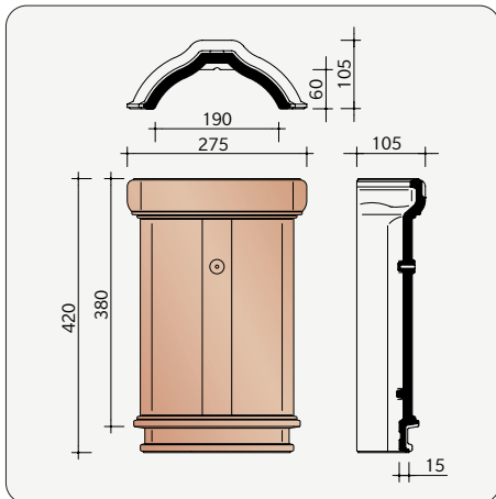
H0001300 2,6 stuks/lm Platte vorst - Noordboom PH
