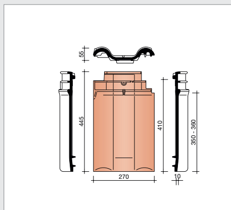
L158050 2,8 stuks/lm Pan met dubbele wel
