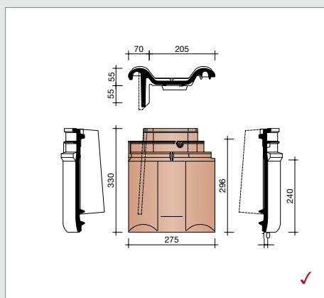
L157000 Linker korte gevelpan
