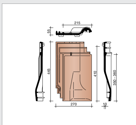
L158610 Ventilatiepan met metalen rooster - 15 cm 2
