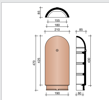
L0001160 Halfronde beginnoordboom - 180 mm
