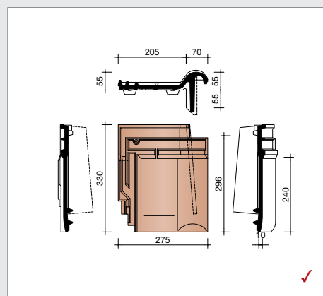
L157010 Rechter korte gevelpan
