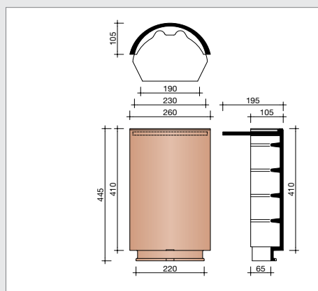
L0001210 Halfronde begin- en eindvorst met kopplaat - 230 mm
