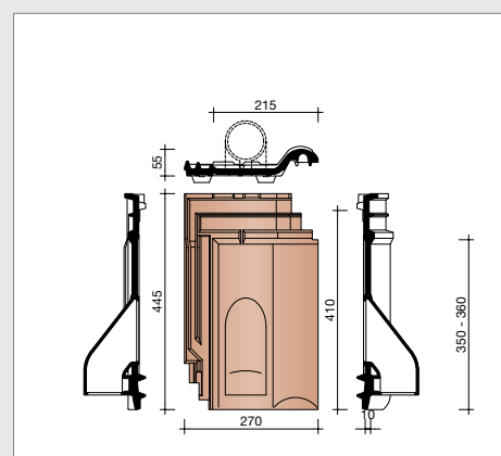
L158958 Kabeldoorvoerpan Ø 60 mm
