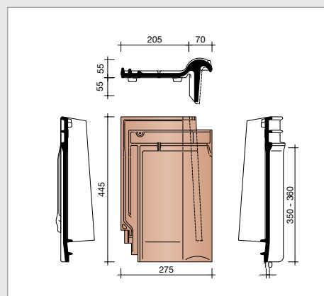
L157090 2,8 stuks/lm Rechter gevelpan
