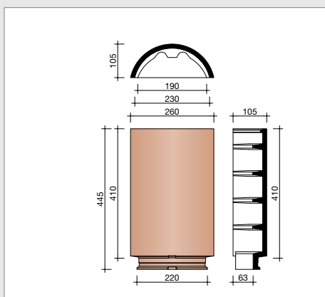
L0001200 2,5 stuks/lm Halfronde vorst - 230 mm
