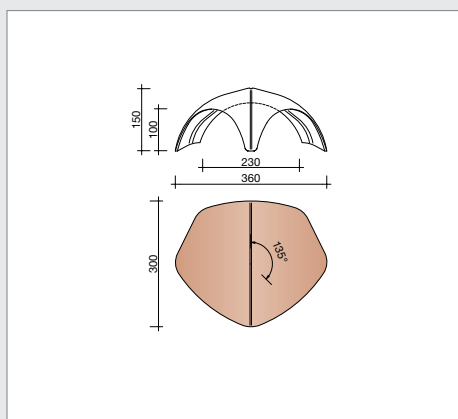
L0005510 Vorstenhoed tussen 1 vorst 1100 en 2 noordbomen 1100
