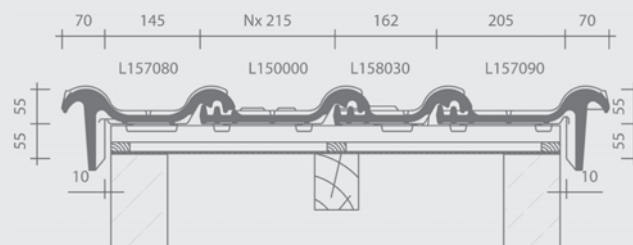
Dwarsdoorsnede dak ter hoogte van gevelpannen
