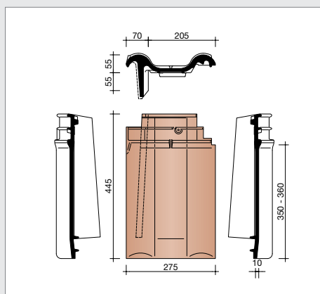
L157080 2,8 stuks/lm Linker gevelpan
