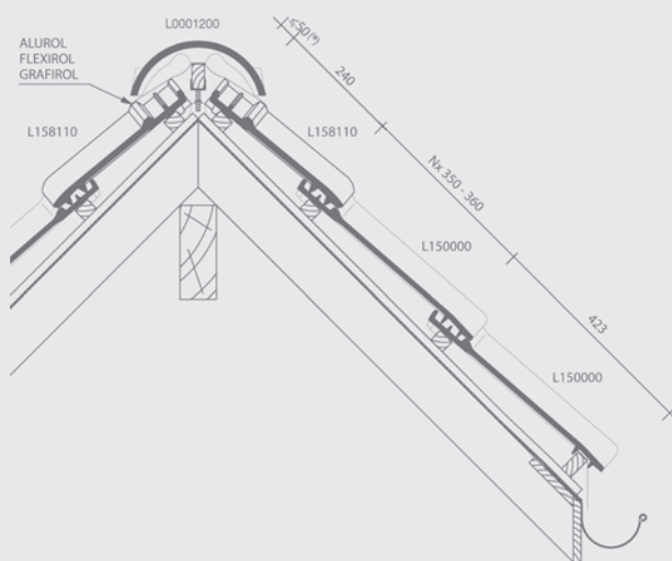
Dwarsdoorsnede dak ter hoogte van vorst
