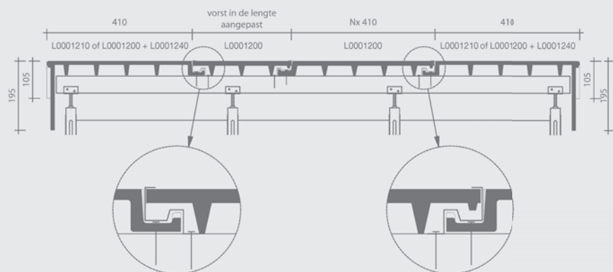
Dwarsdoorsnede dak ter hoogte van vorst
