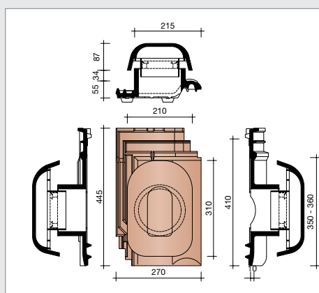
L158728 Kit kokerpan + kapje Ø 125 mm + aansluitingsmodule + reductorstuk
