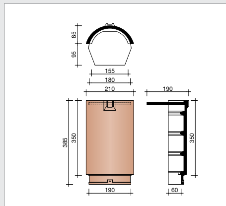
L0001110 Halfronde begin- en eindvorst met kopplaat - 180 mm
