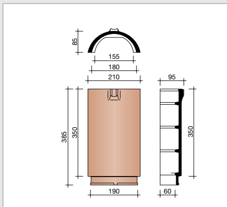
L0001100 3 stuks/lm Halfronde vorst - noordboom - 180 mm
