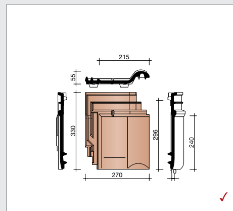
L158110 4,65 stuks/lm Korte pan
