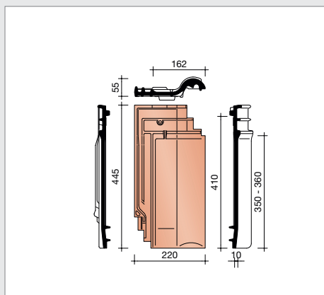
L158030 2,8 stuks/lm 3/4 pan
