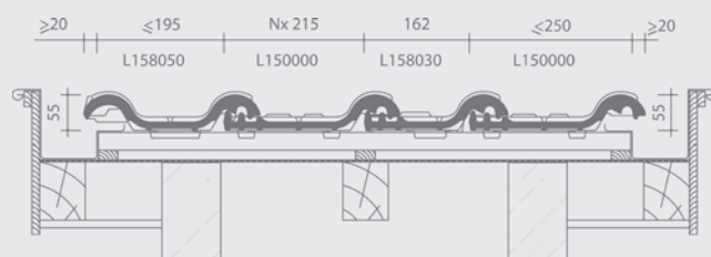
Dwarsdoorsnede dak ter hoogte van pan met dubbele wel
