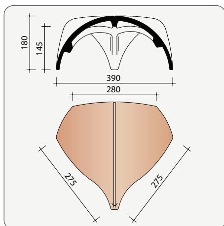
H0005230 Vorstenhoed W2 PV/PH/PI voor 1 vorst en 2 noordbomen
