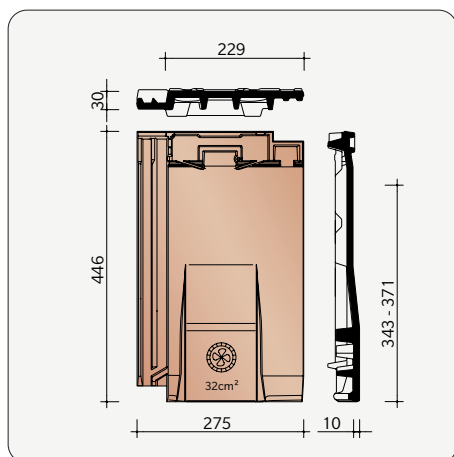
HMIK8610 Ventilatiepan - 32 cm 2
