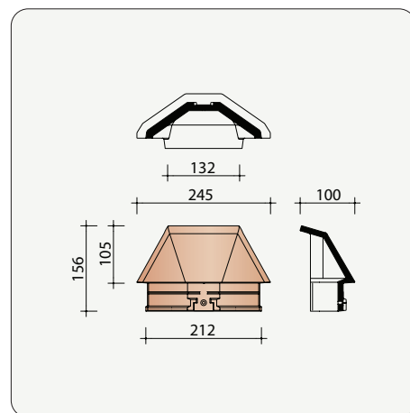
H0002860 Hoekige beginnoordboom PI
