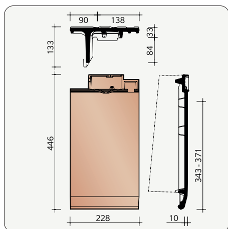
HMIK7081 2,7 stuks/lm Linker gevelpan Duits model
