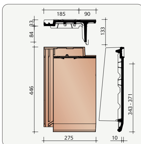
HMIK7091 2,7 stuks/lm Rechter gevelpan Duits model
