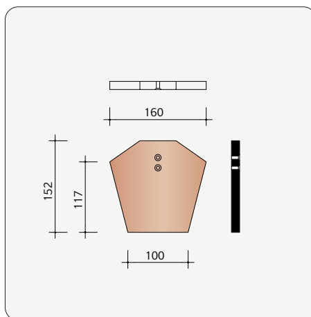
H0002840 Kopplaat voor hoekige vorst PI
