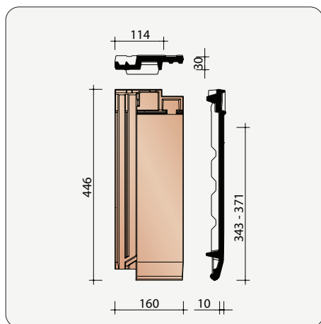
HMIK8010 1,35 stuks/lm kruisgewijs Halve pan 2,7 stuks/lm recht
