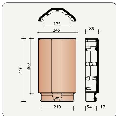
H0002800 2,8 stuks/lm Hoekige vorst - Noordboom PI
