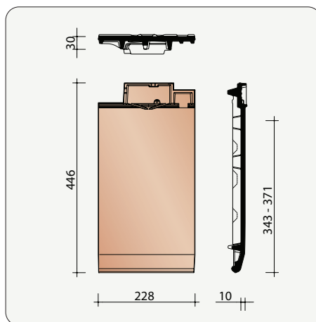
HMIK8045 2,7 stuks/lm Pan zonder zijsluiting
