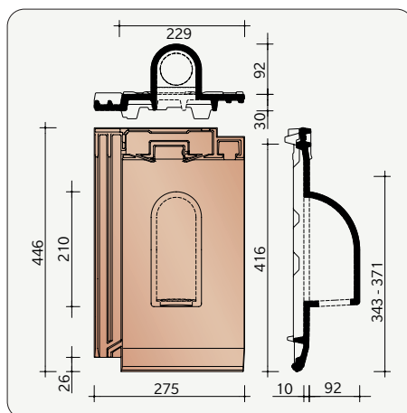
HMIK8958 Kabeldoorvoerpan (Solar) + onderdakadapter
