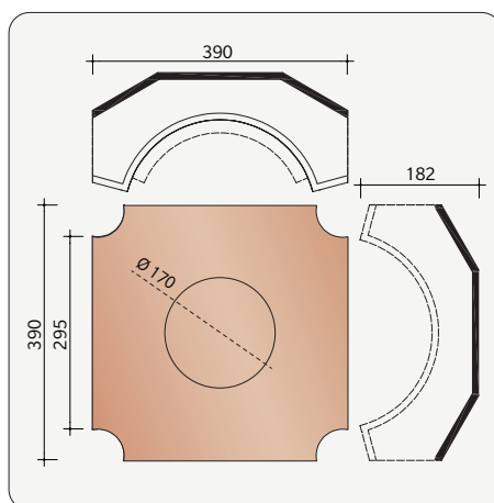
H0005240 Vorstenhoed W2 PV/PH/PI voor 4 noordbomen
