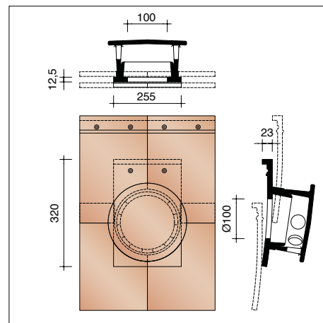
PPLA8961 Kit tuile à douille Ø 100 mm + mitron - 95 cm² + module de connexion
