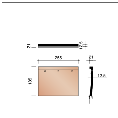
PPLA8110 4 pièces/m crt Tuile raccourcie
