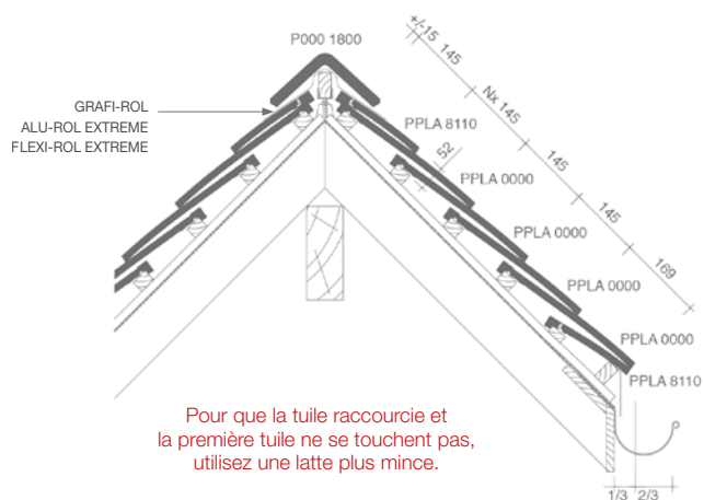
PLAN DE POSE LONGITUDINALE DE LA TOITURE AU NIVEAU DE LA FAÎTIÈRE 1800
