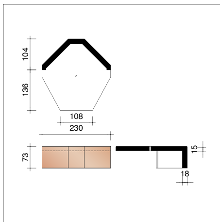
P0002840 Fronton pour faîtière angulaire sans emboîtement
