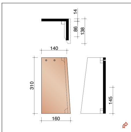
PPLA7130 3,5 pièces/m crt Demi-tuile de rive droite spéciale
