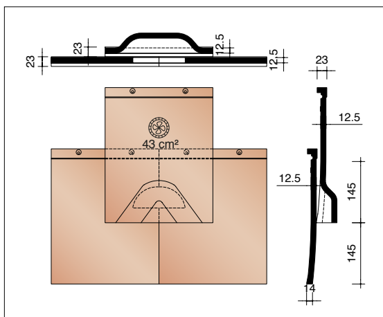
PPLA8611 Kit de ventilation avec grille - 43 cm²
