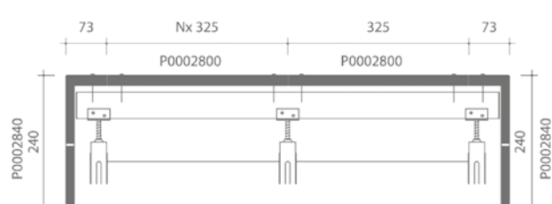
PLAN DE POSE TRANSVERSALE DE LA TOITURE AU NIVEAU DE LA FAÎTIÈRE 2800
