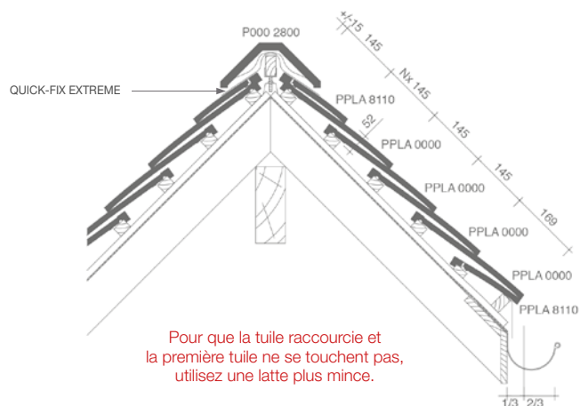
PLAN DE POSE LONGITUDINALE DE LA TOITURE AU NIVEAU DE LA FAÎTIÈRE 2800 - AVEC QUICK-FIX EXTREME
