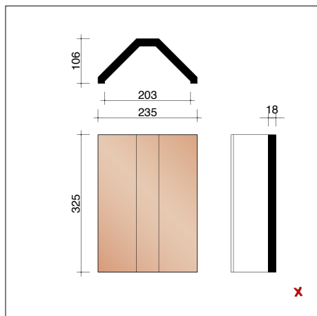
P0002800 3 pièces/m crt Faîtière angulaire sans emboîtement
