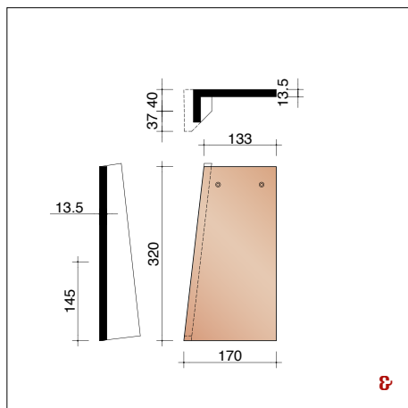
PPLA8800 3,5 pièces/m crt Pièce d'angle gauche (bardage)
