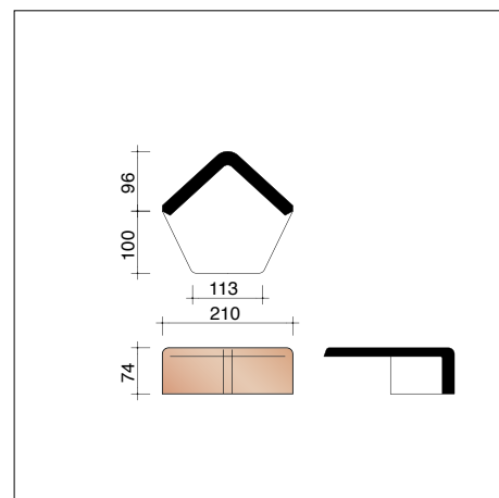
P0001840 Fronton pour faîtière angulaire
