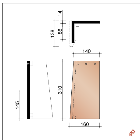
PPLA7120 3,5 pièces/m crt Demi-tuile de rive gauche spéciale
