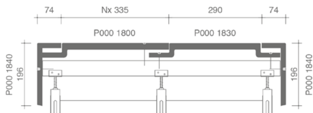
PLAN DE POSE TRANSVERSALE DE LA TOITURE AU NIVEAU DE LA FAÎTIÈRE 1800
